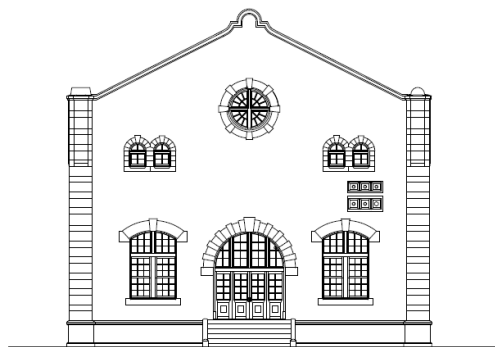
西立面図
