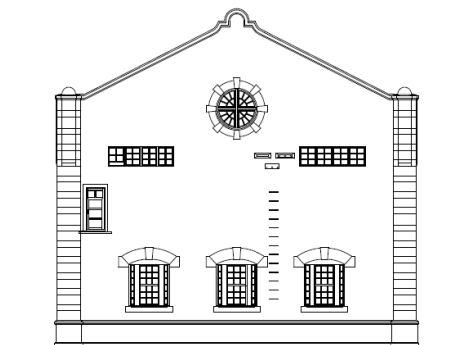
東立面図
