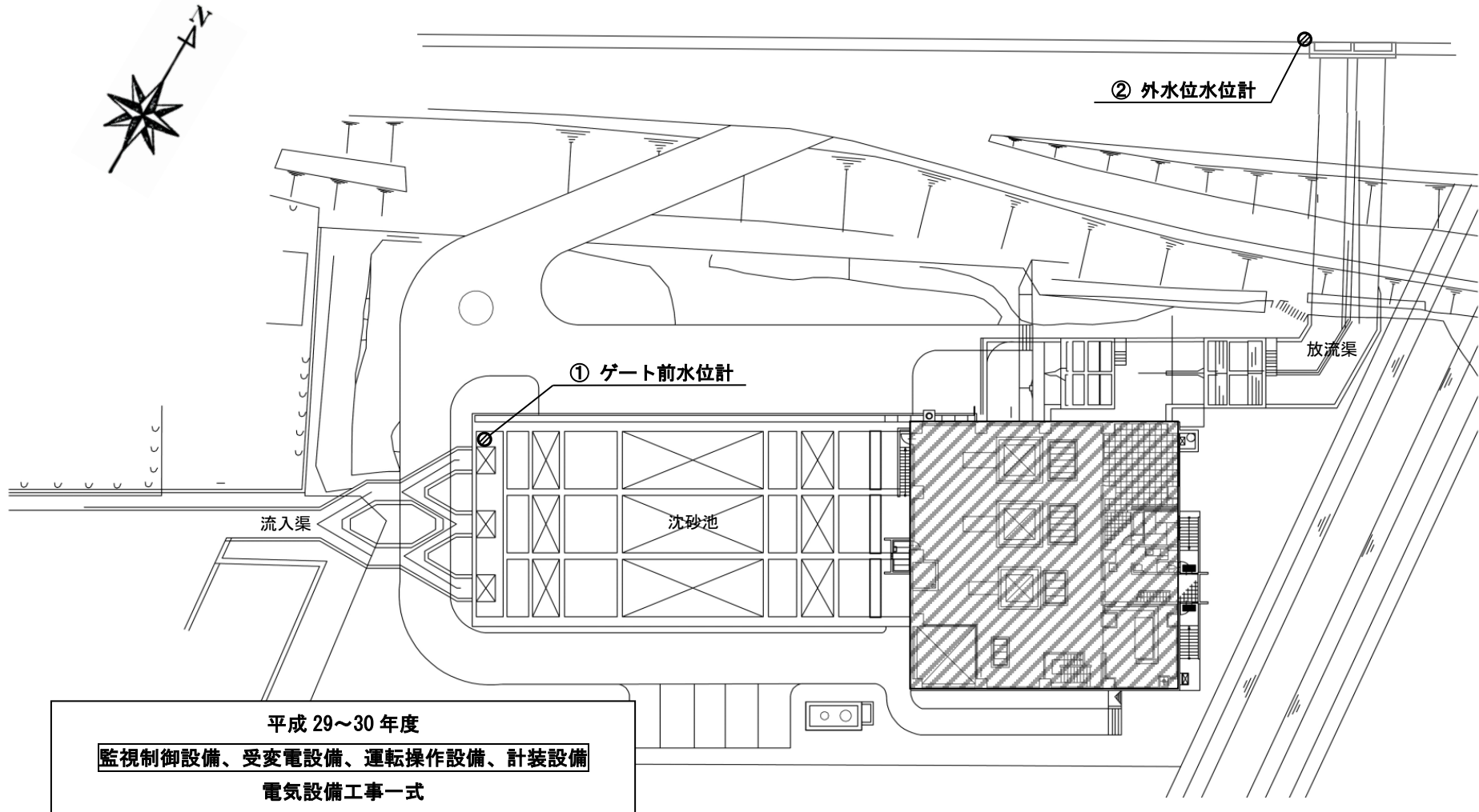
松神子雨水ポンプ場 平面図
