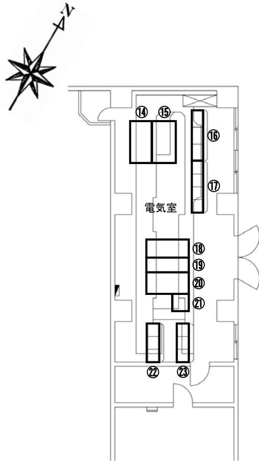
松神子雨水ポンプ場3階 配置図
