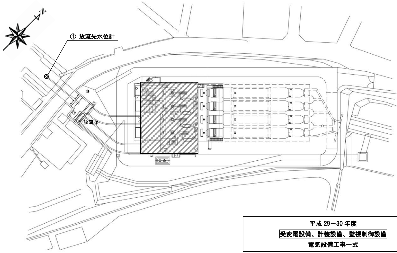
沢津雨水ポンプ場 平面図
