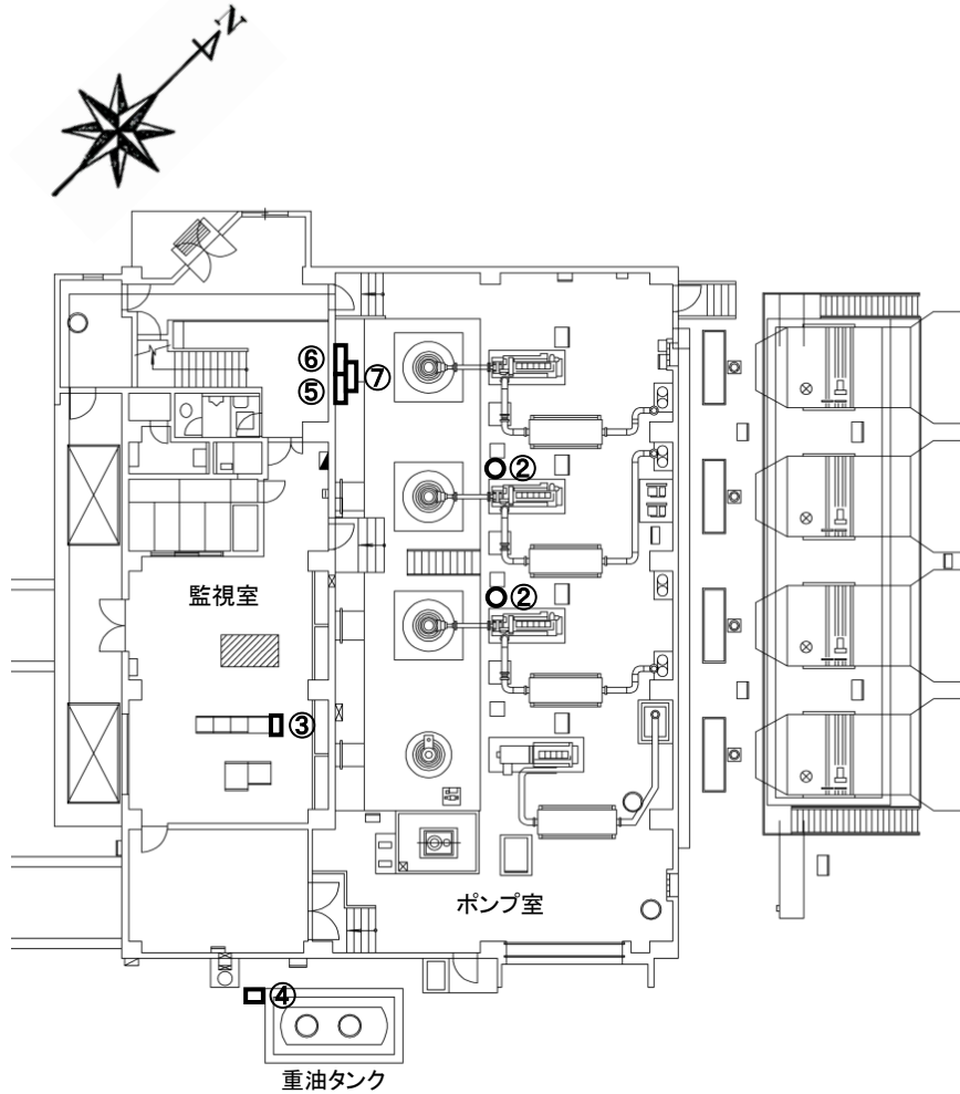
沢津雨水ポンプ場 1階 配置図
