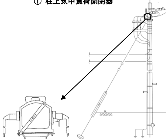
① 柱上気中負荷開閉器
