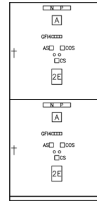
④ No. 1・No. 2コンデンサ盤
