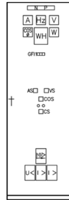
③ 受電盤
