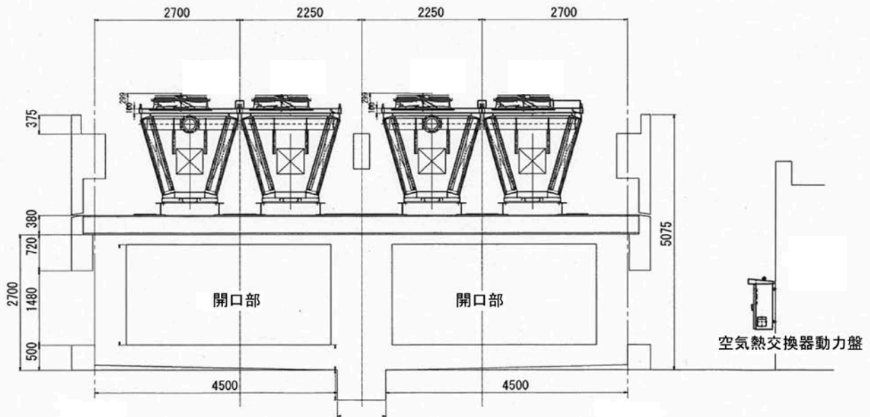
庁舎 屋上施工図
