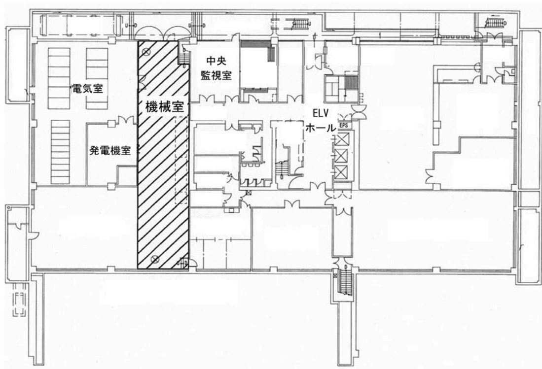
庁舎 地下1階平面図
