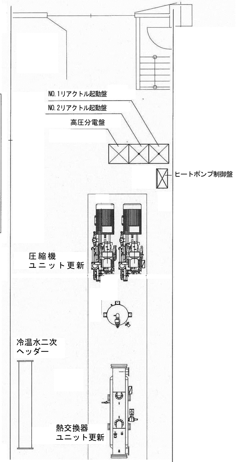
庁舎 地下1階機械室施工平面図
