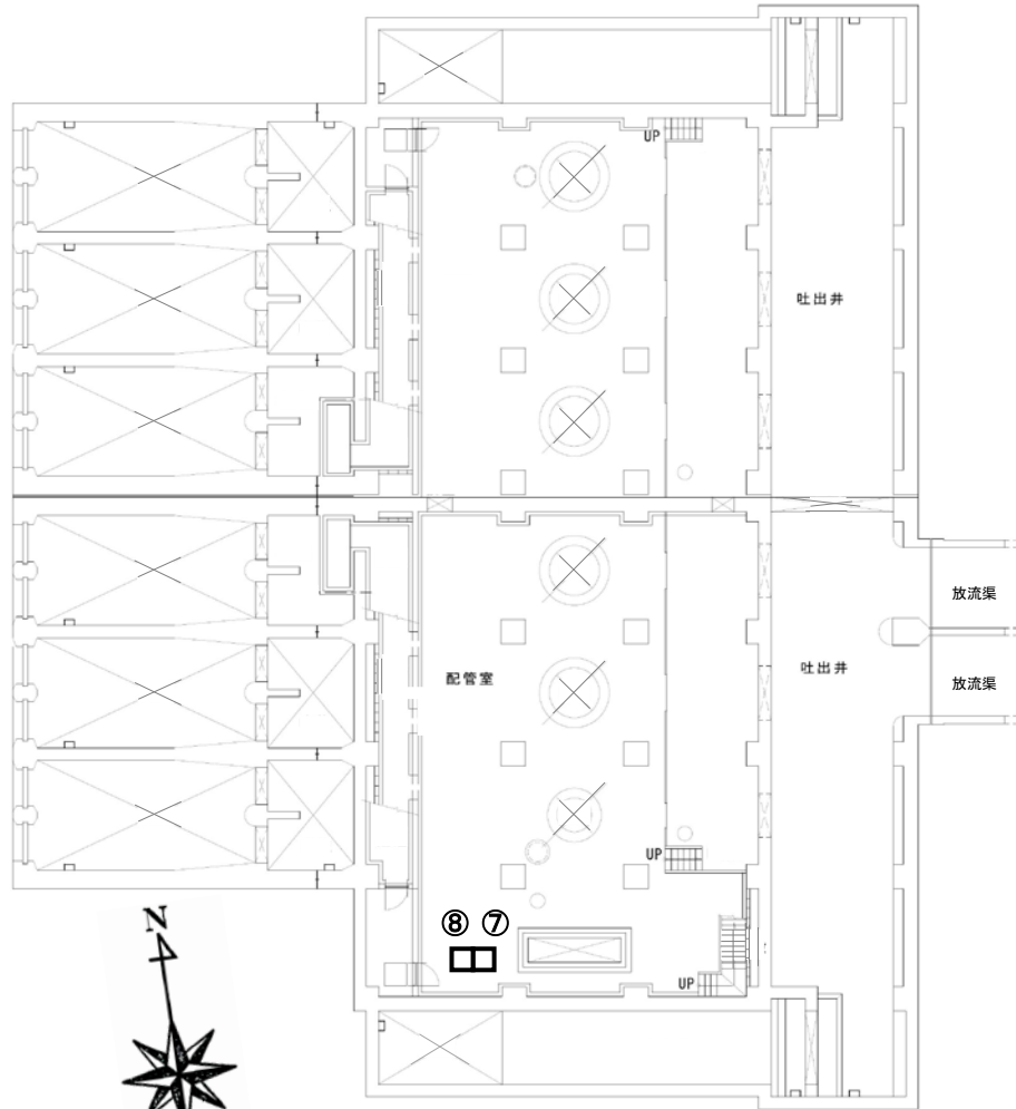
地下1階 配置図
