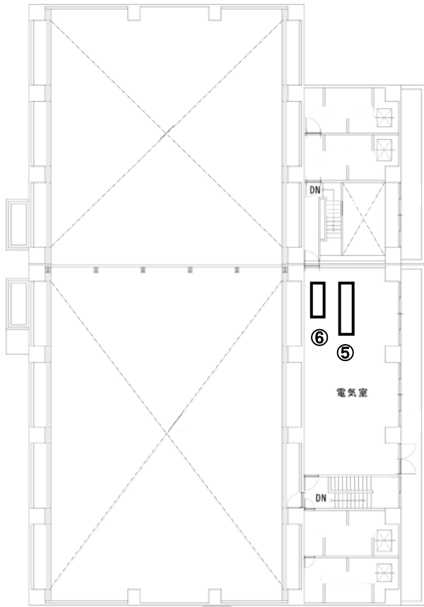
2階 配置図
