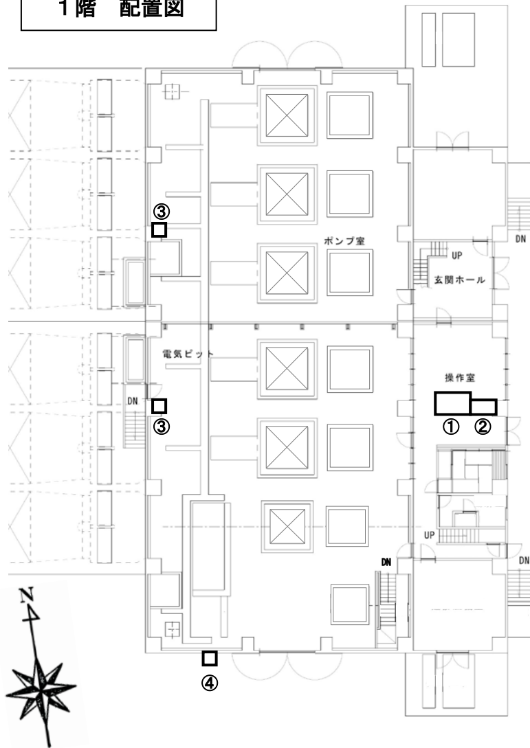
1階 配置図
